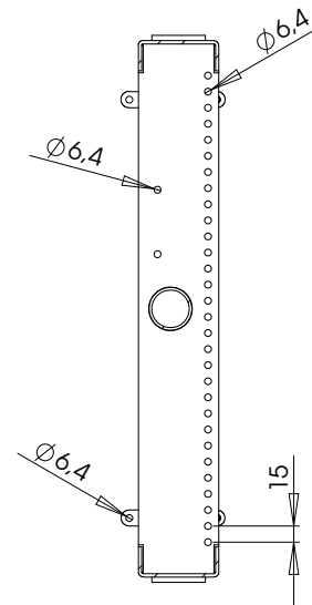
SCHNITT A-A
